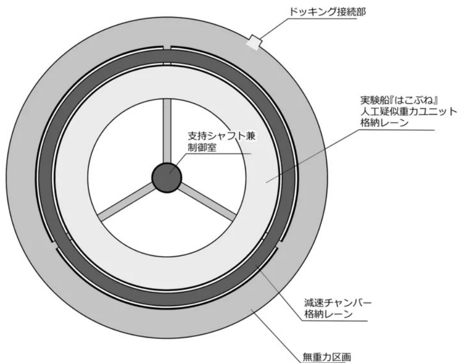
月軌道ステーション<スペースアンカーファースト> 垂直方向から見た簡易模式図
